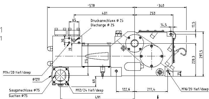
Fußmaßzeichnung Footprint
