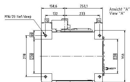
Fußmaßzeichnung Footprint
