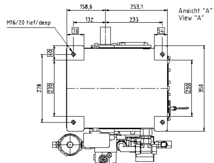
Fußabdruck Footprint
