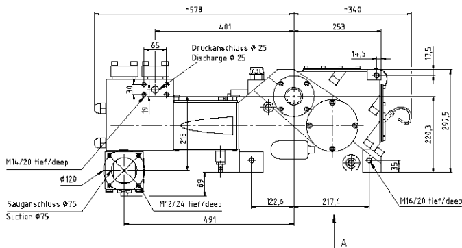
Fußabdruck Footprint
